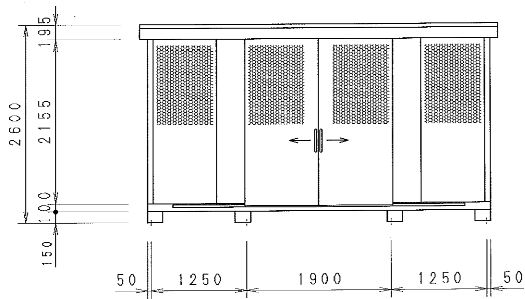
正面図
