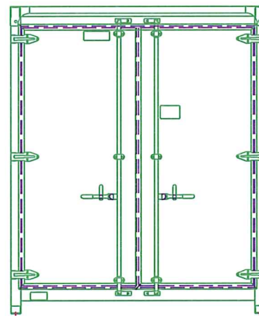
D立面図
