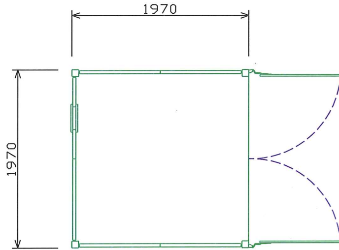
平面図
