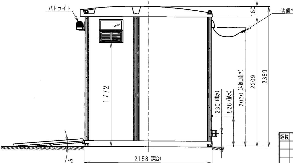
側面図
