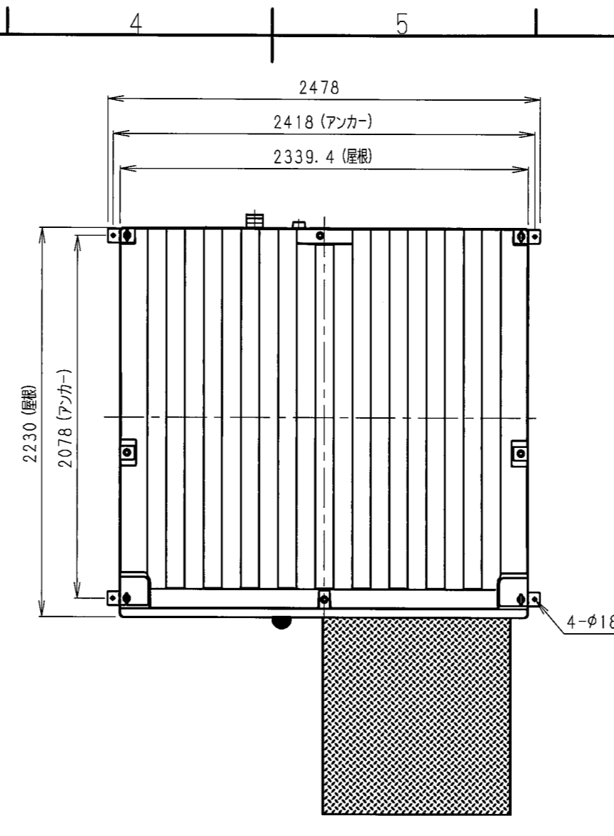
屋根伏図
