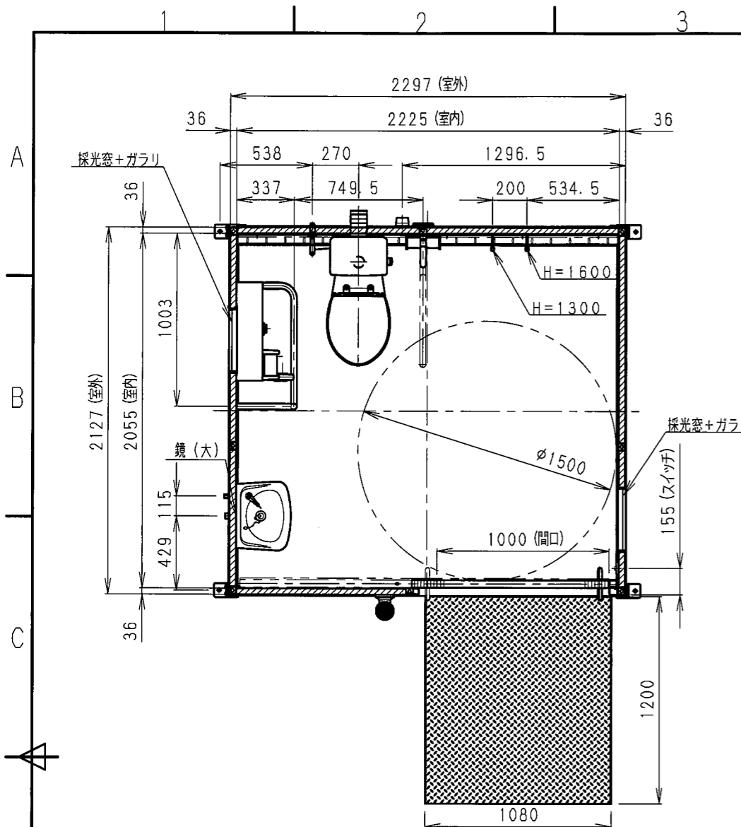
平面図
