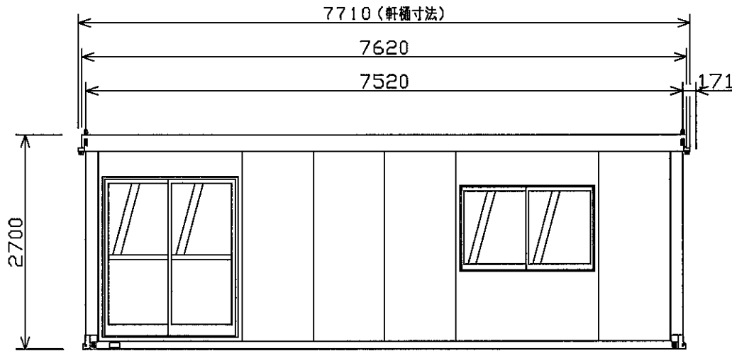
A 立面図
