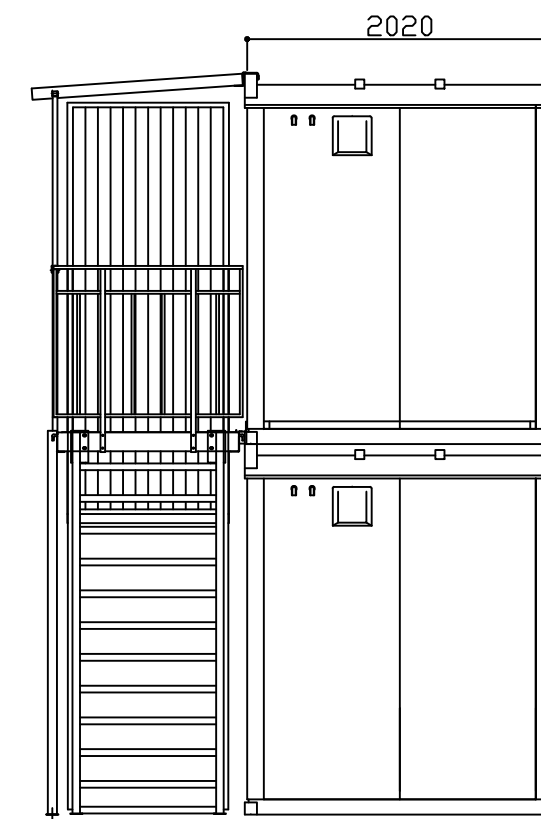
D 立面図 S=1/50
