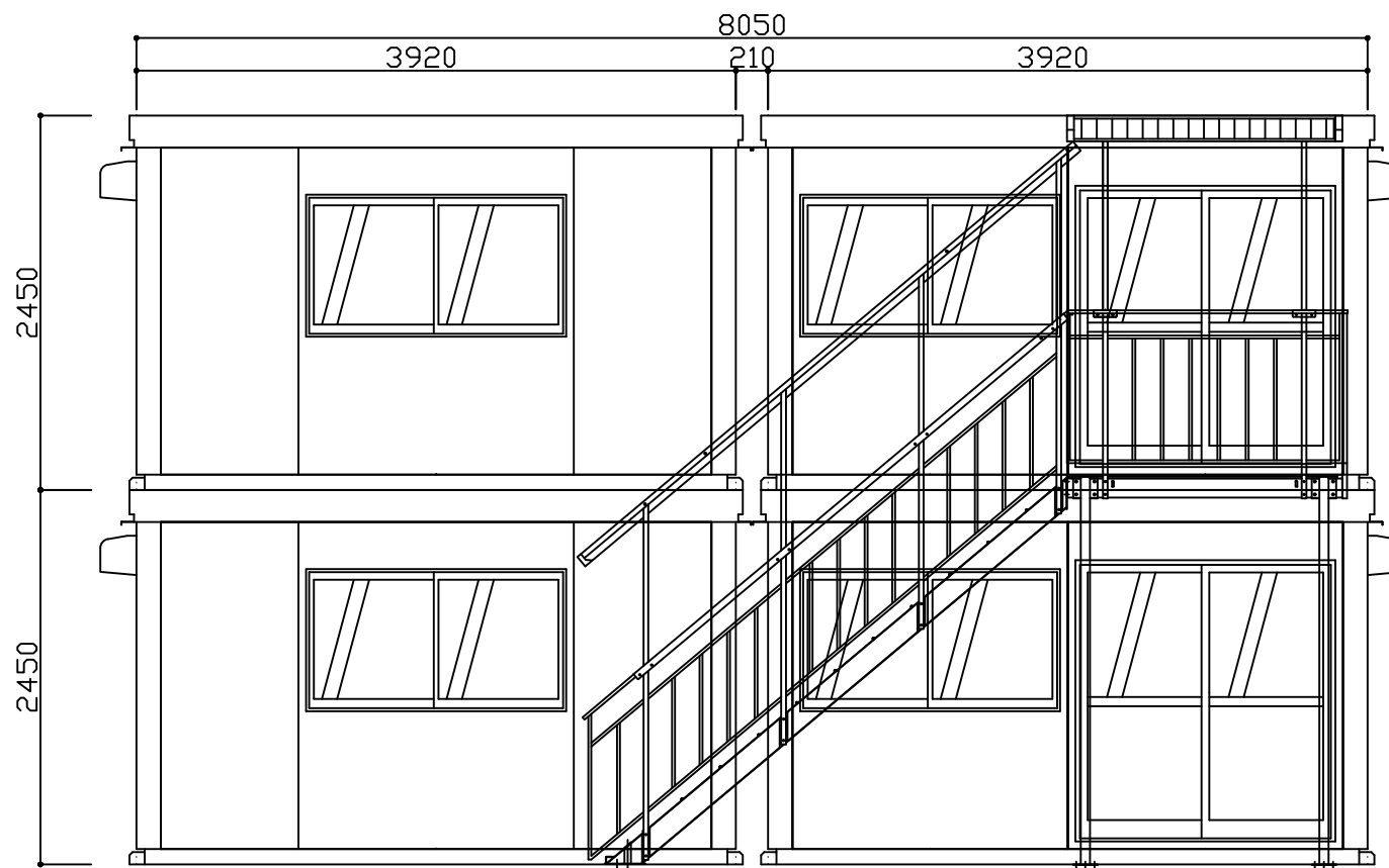
A 立面図 S=1/50
