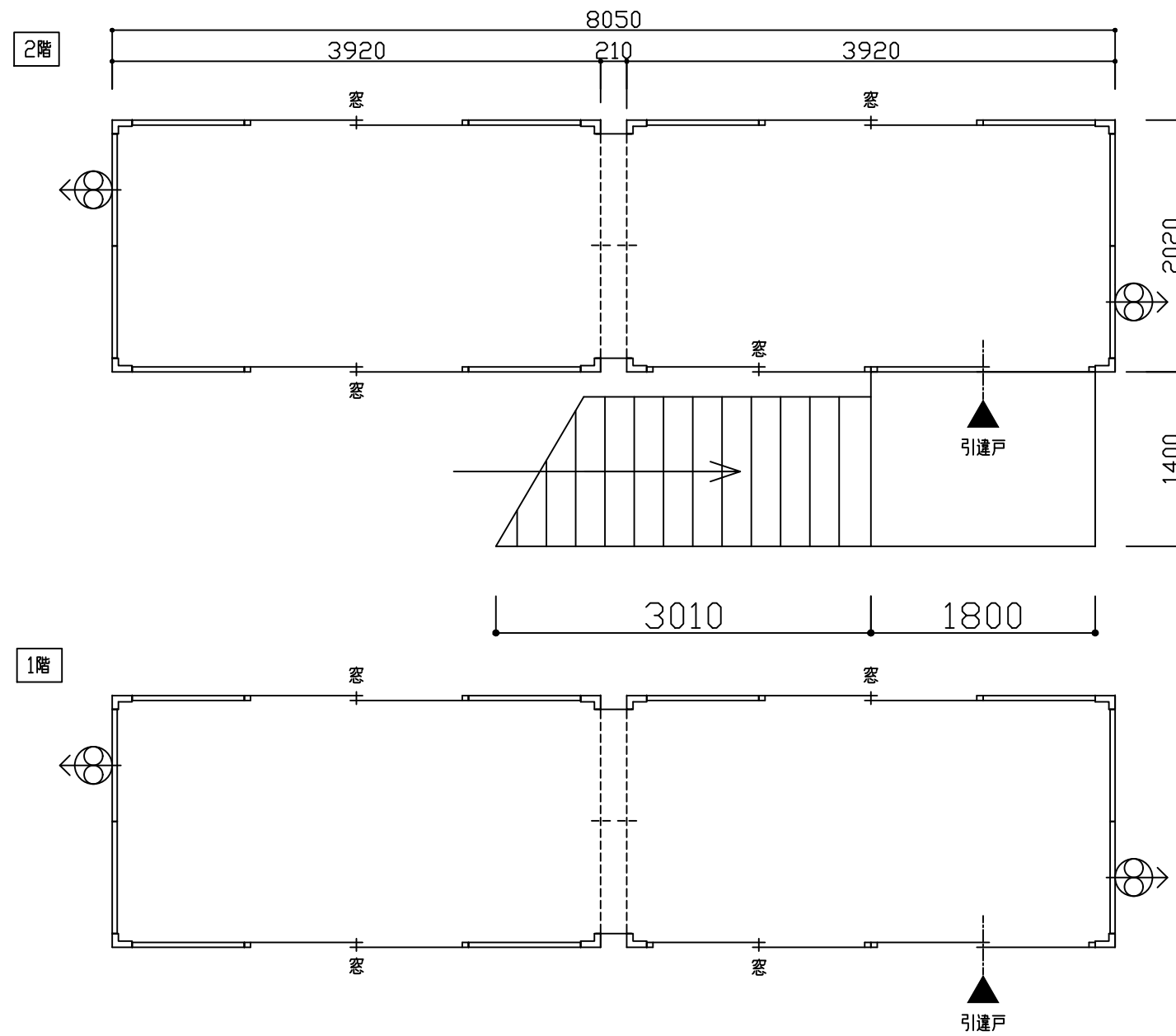
平面図 S=1/50
