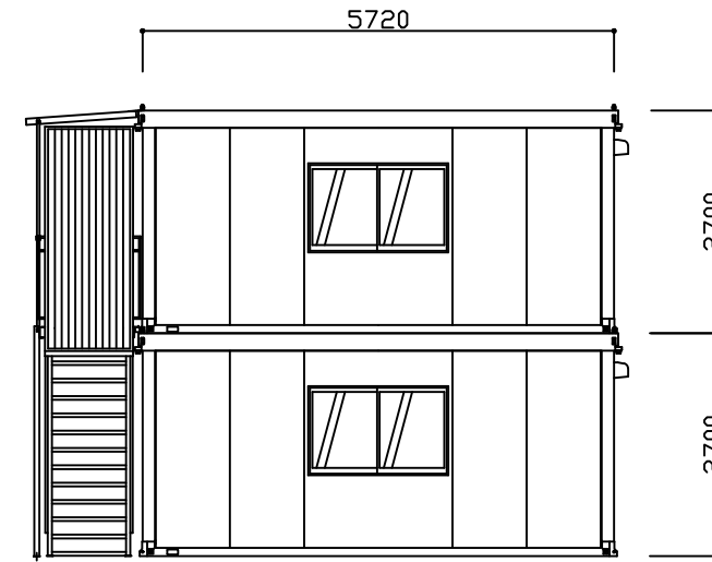
D 立面図 S=1/100
