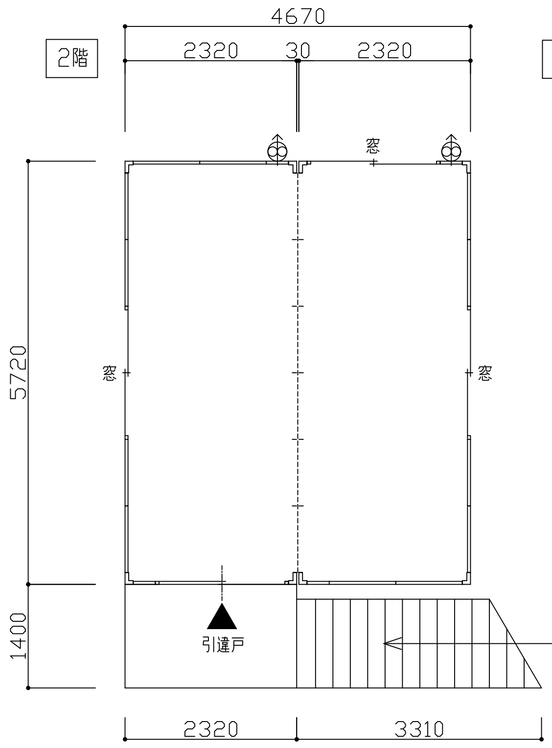
平面図 S=1/50
