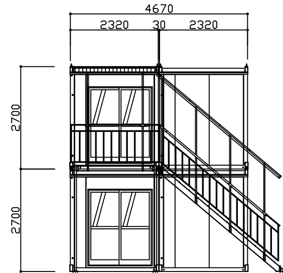
A 立面図 S=1/100
