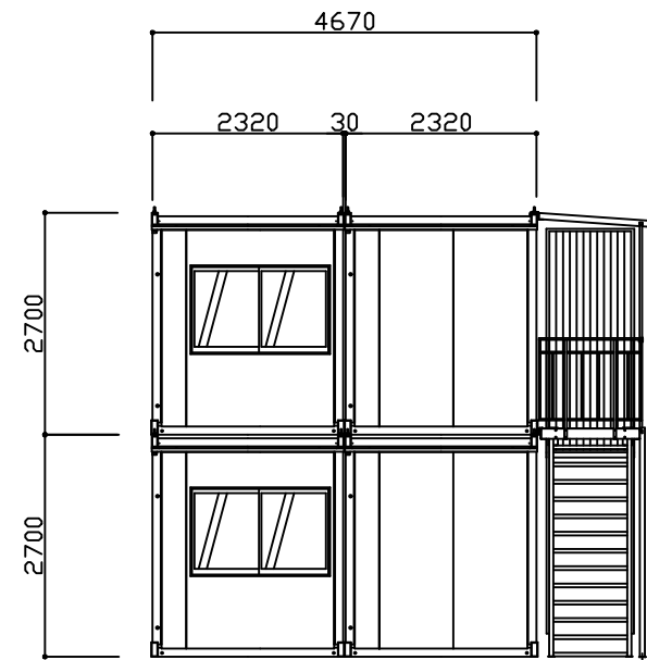
A 立面図 S=1/100
