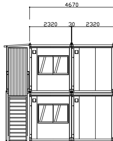
C 立面図 S=1/100
