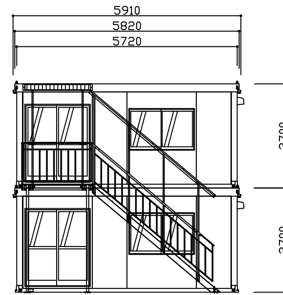
D 立面図 S=1/100
