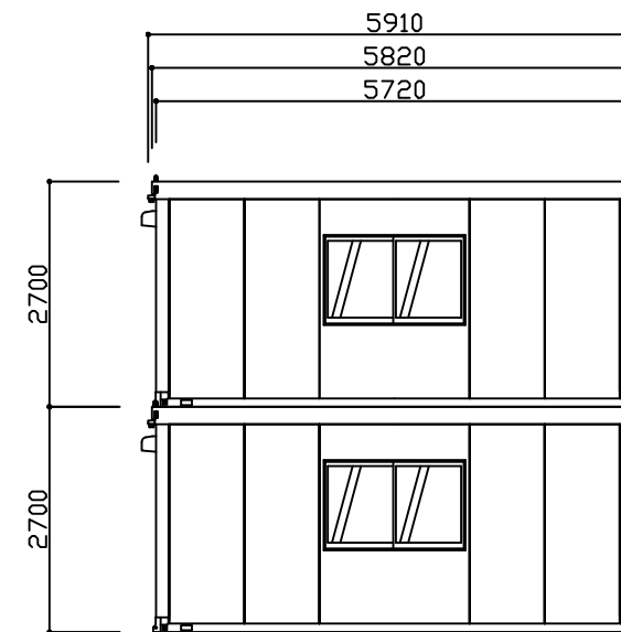
B 立面図 S=1/100
