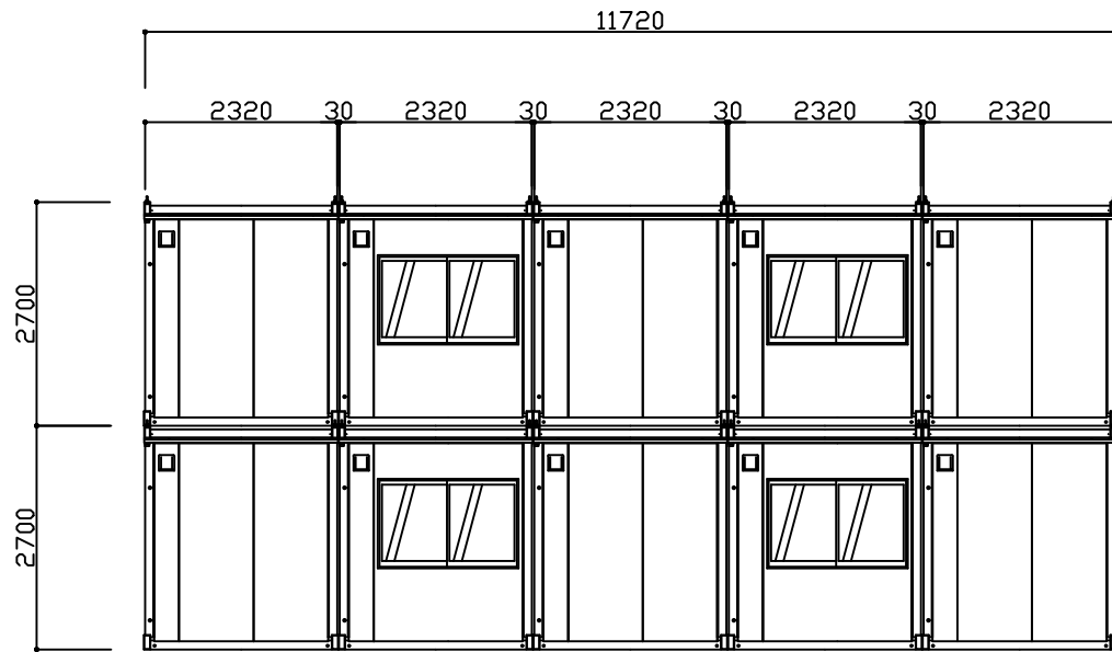
C 立面図 S=1/100
