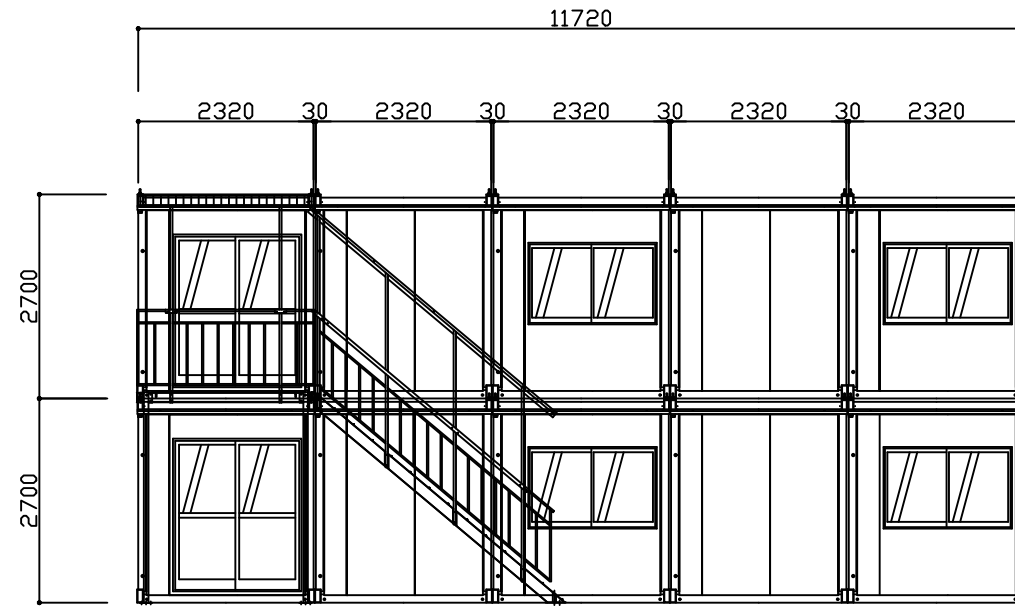
A 立面図 S=1/100
