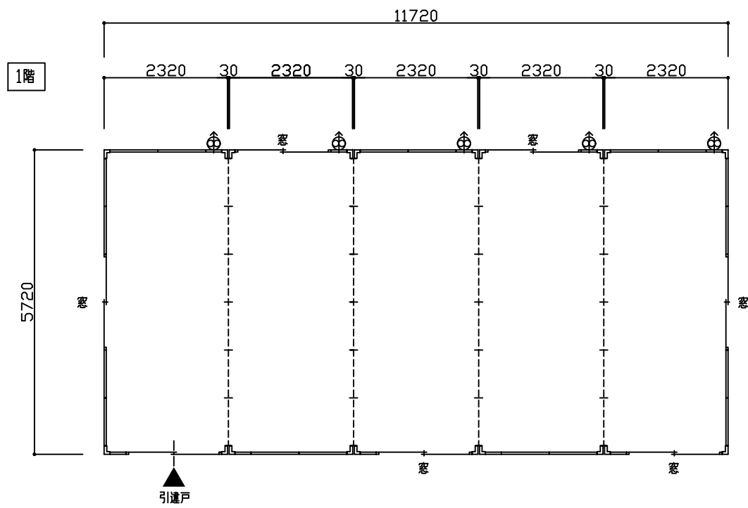
平面図 S=1/100
