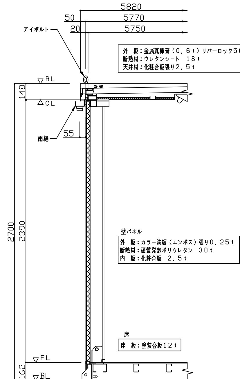
矩 計 図 S=1/20
