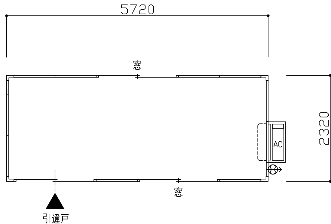
平面図 S=1/50
