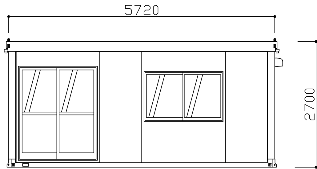
A 立面図 S=1/50
