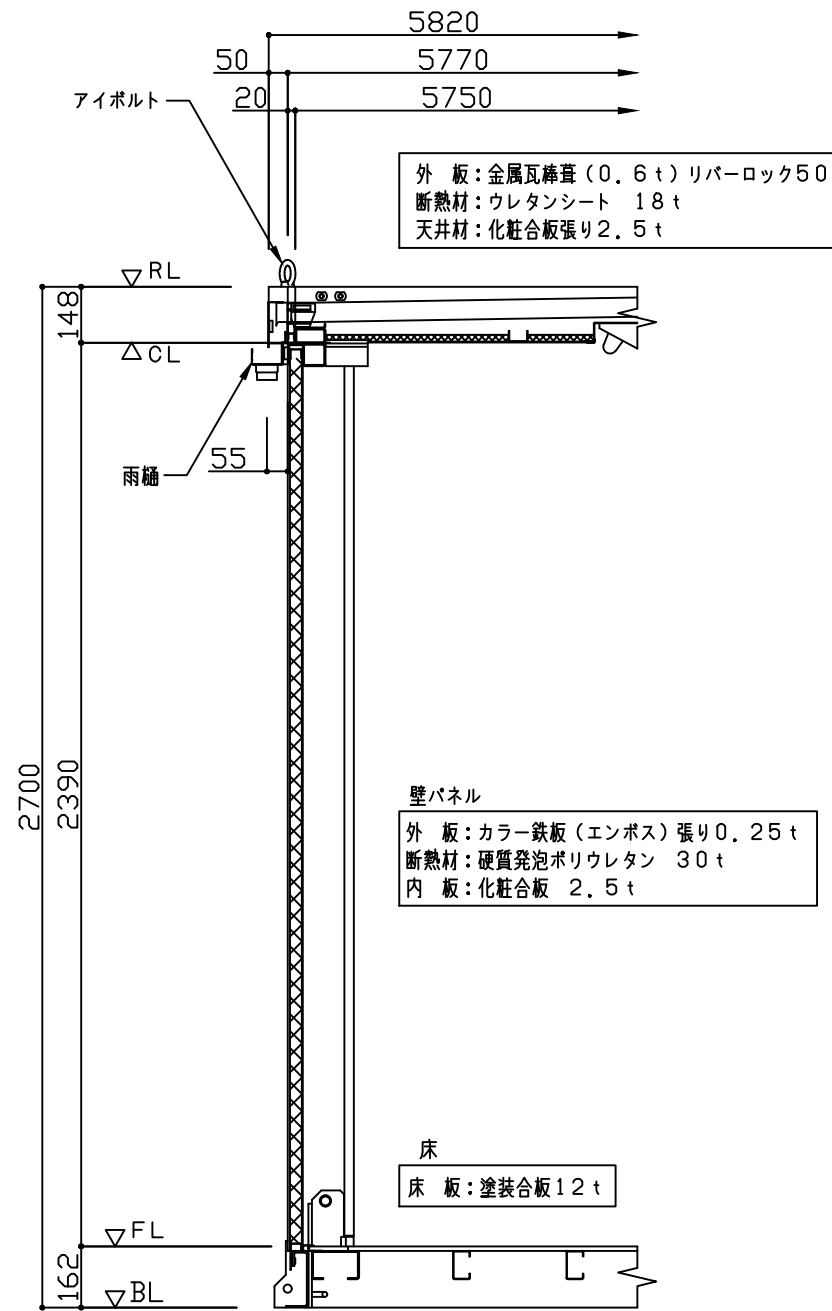
矩計図 S=1/20
