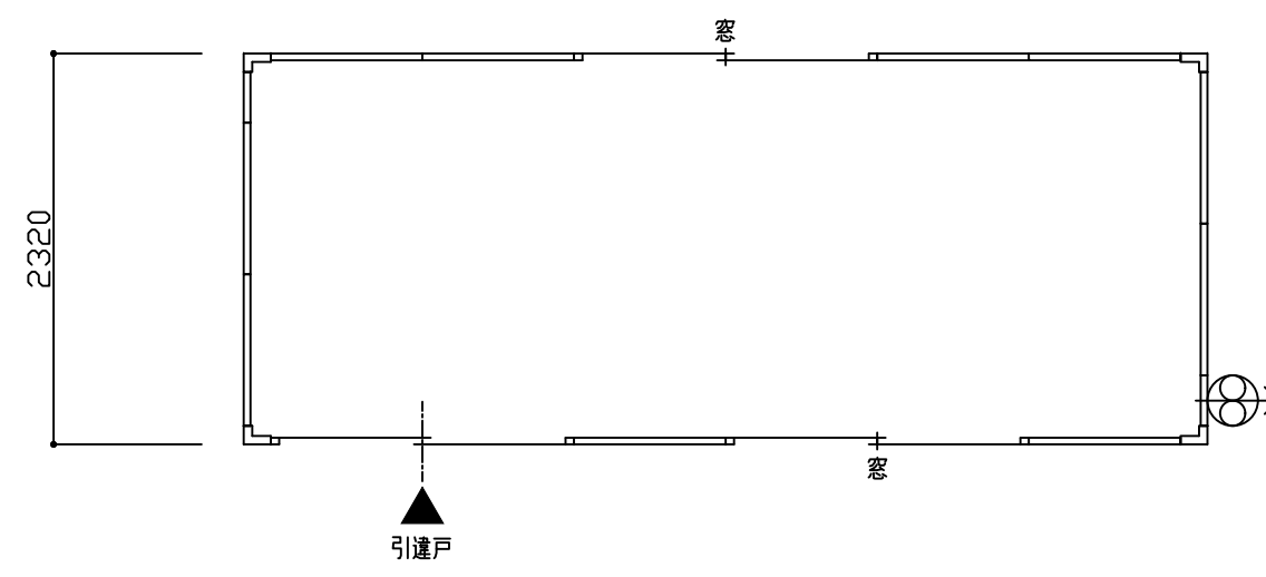
平面図 S=1/50
