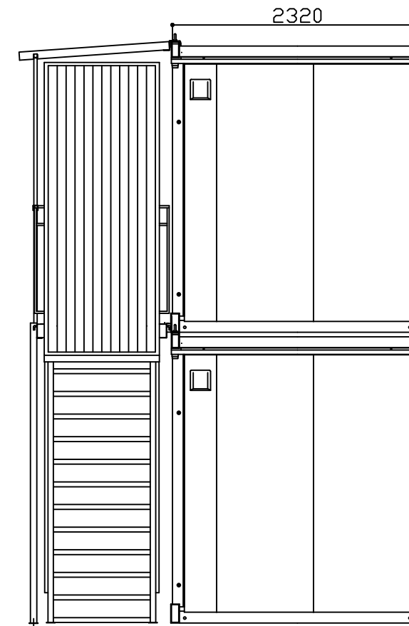
D 立面図 S=1/50
