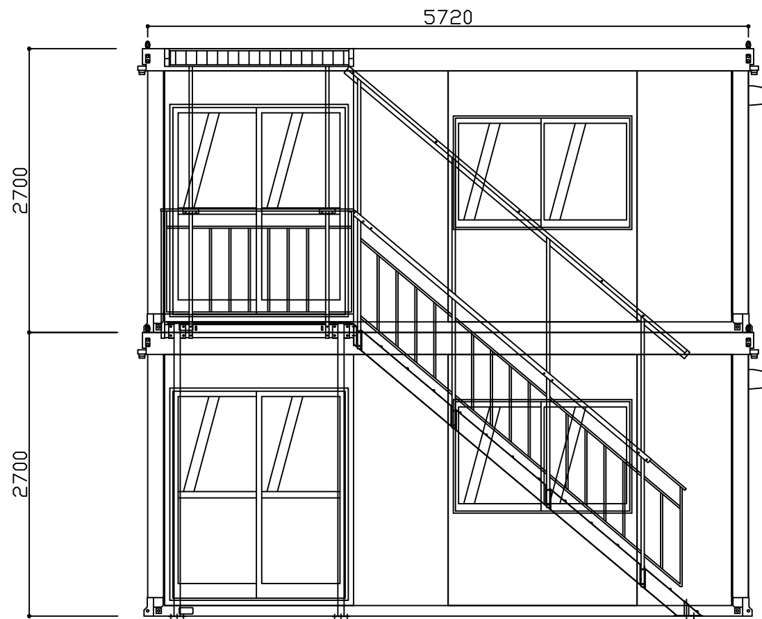
A 立面図 S=1/50
