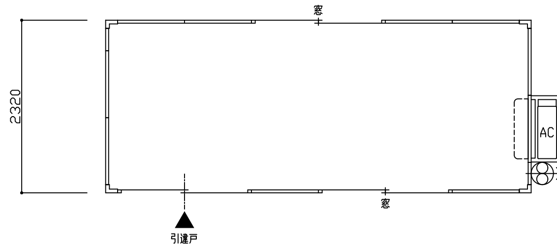
平面図 S=1/50
