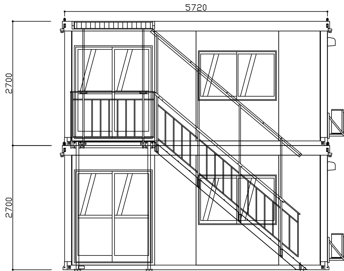
A 立面図 S=1/50
