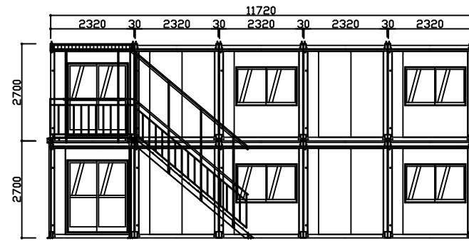
A 立面図 S=1/150
