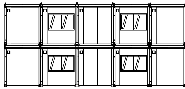
C 立面図 S=1/150
