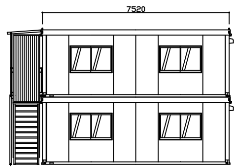
D 立面図 S=1/150
